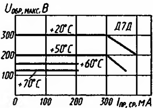
Зависимости допустимого обратного напряжения от тока
