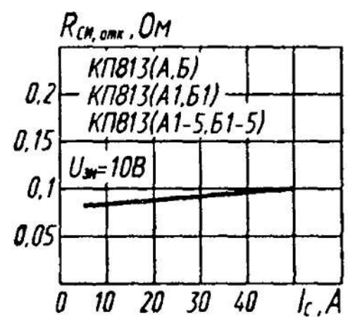
Зависимость сопротивления сток—исток от тока стока
